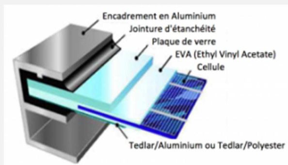
Figure 8 : Composition d'un panneau photovoltaïque
