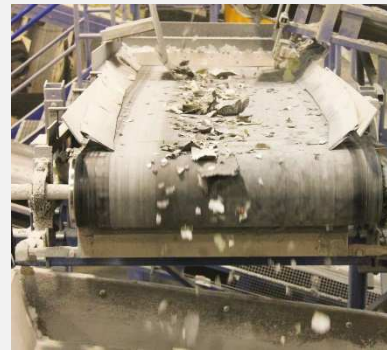
Figure 10 : Panneau photovoltaïque broyé (© PV CYCLE) 9
